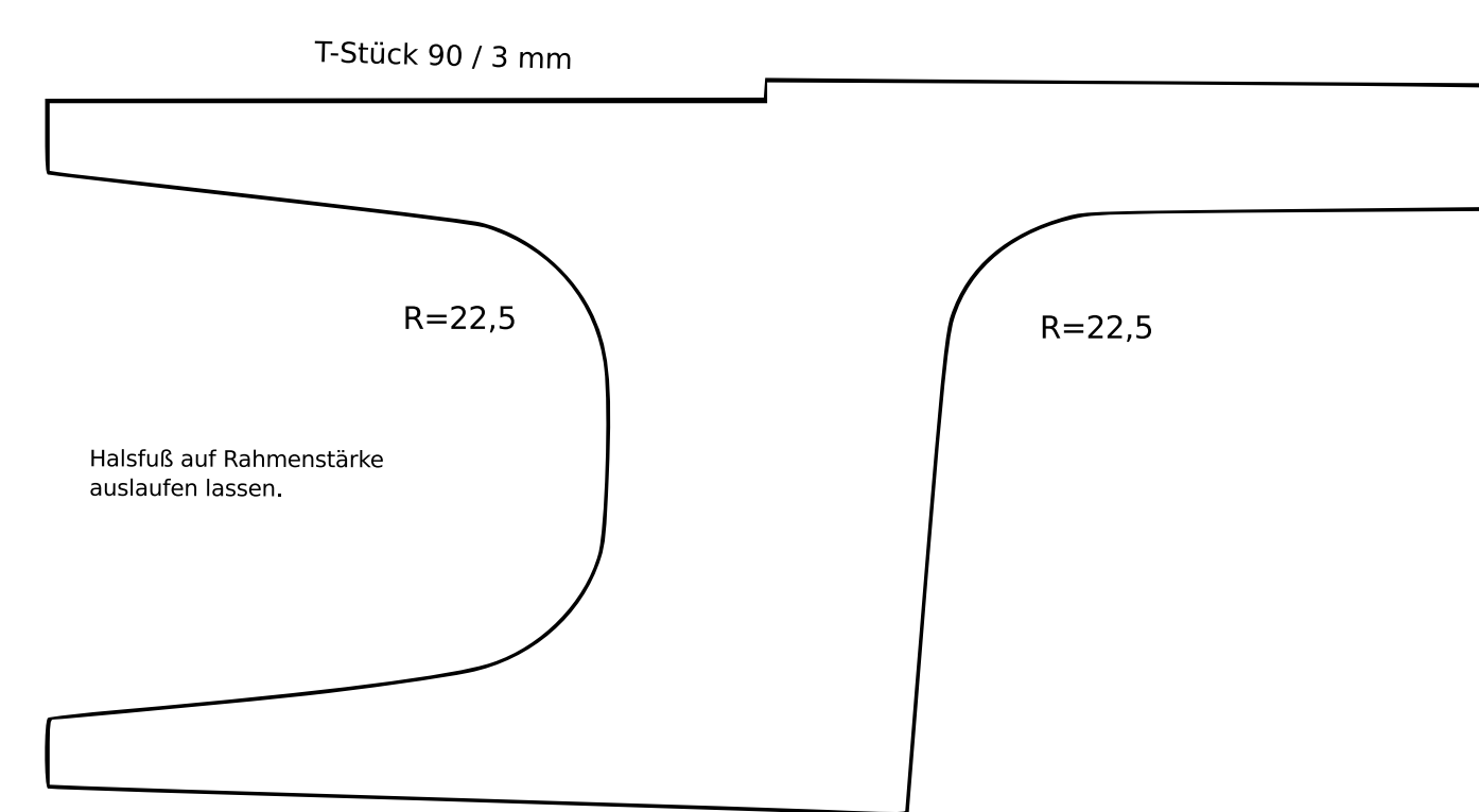
Breite T-Stück Boden 285 mm, Höhe 108 mm Rahmen im Bereich der T-Stücke um Materialstärke reduzieren.
