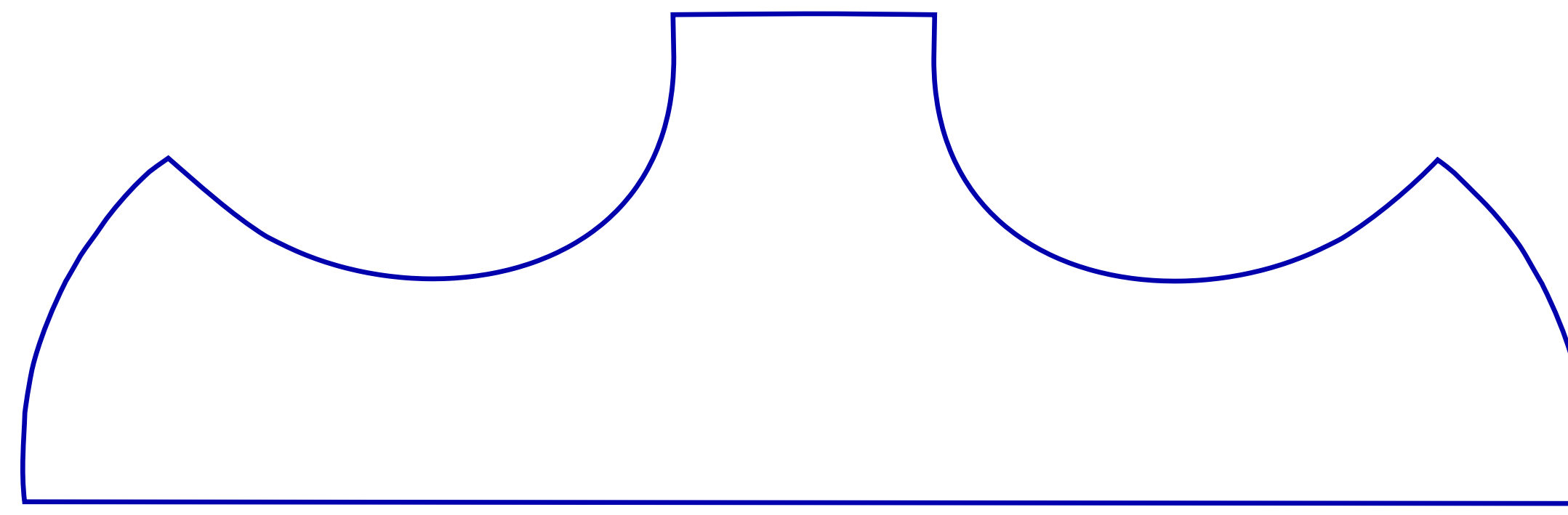
Breite T-Stück Decke 285 mm, Höhe 90 mm, Dicke 3 -4 mm 3-fach Furnierlaminat
