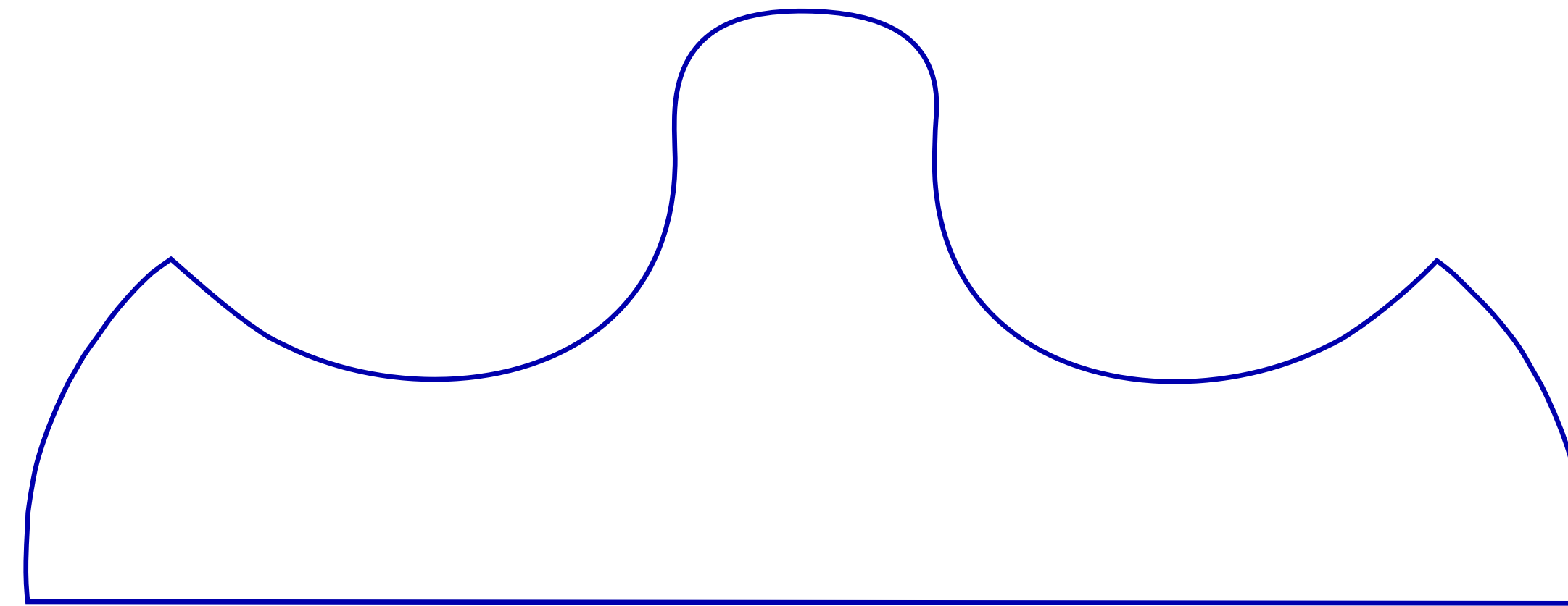
Breite T-Stück Decke 285 mm, Höhe 90 mm, Dicke 3 -4 mm 3-fach Furnierlaminat
