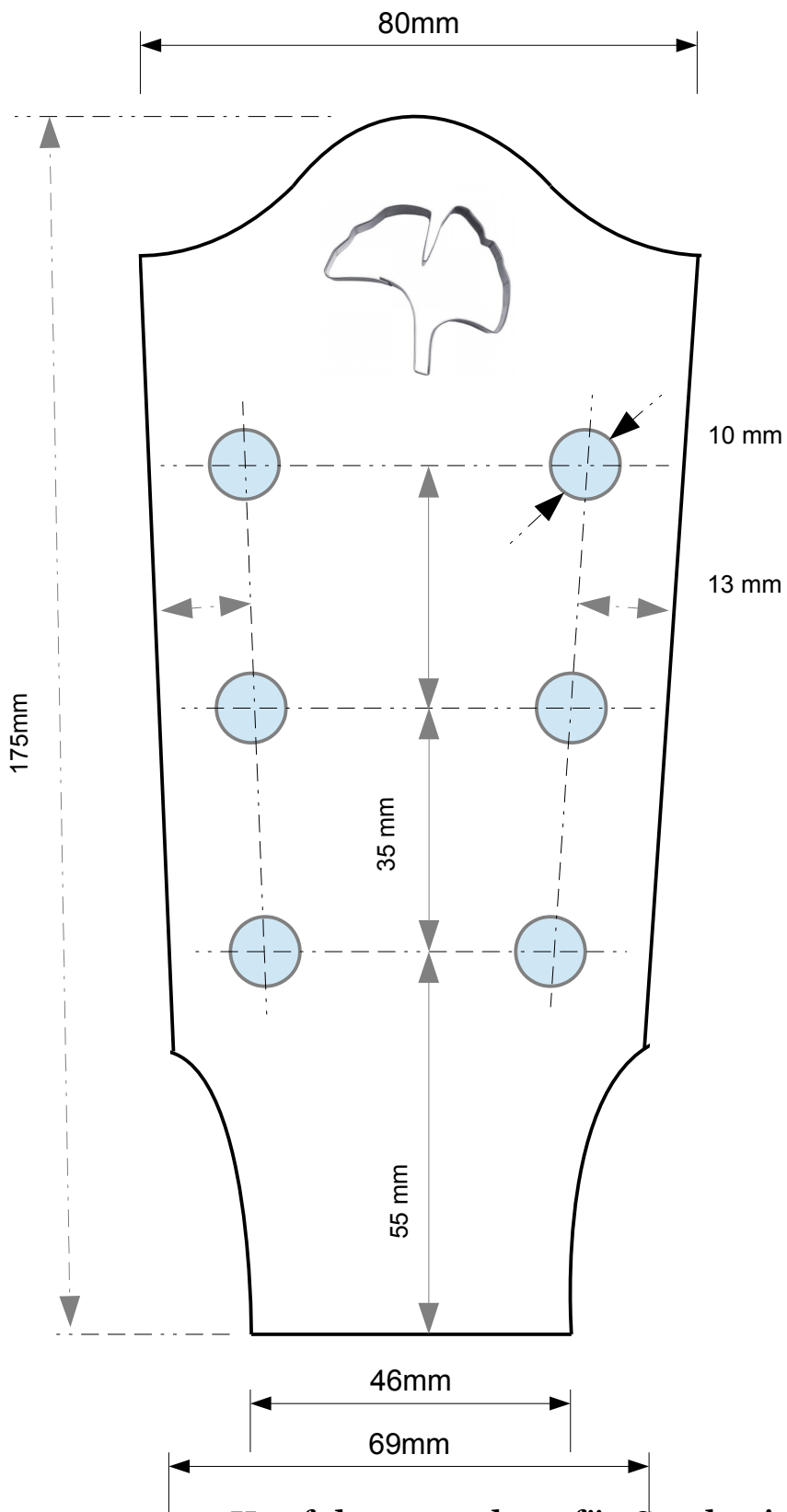
Kopfplattenvorlage für Steelstring Gitarre Lutz Splettstösser 2014 Maßstab 1:1 (beim Drucken bitte auf Originalgröße achten)
